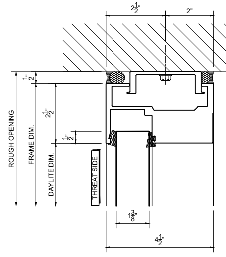
7 HEAD DETAIL SCALE: 3" = 1'-0"
