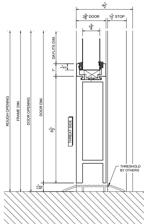
2 DOOR BOTTOM DETAIL SCALE: 3" = 1'-0"
