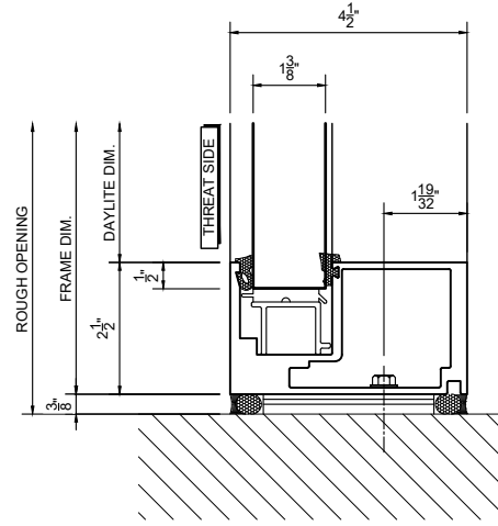
9 SILL DETAIL SCALE: 3" = 1'-0"
