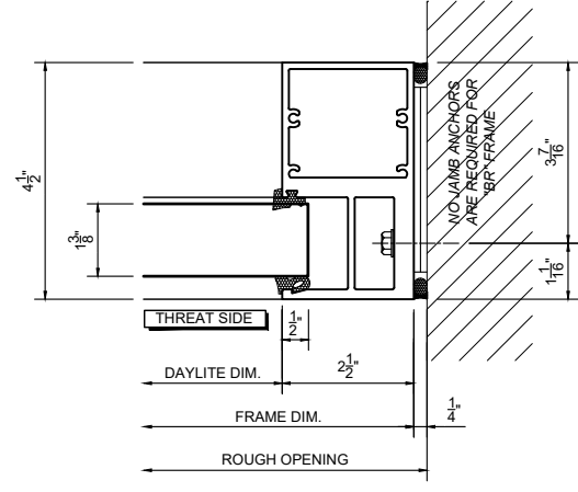
10 JAMB DETAIL SCALE: 3" = 1'-0"
