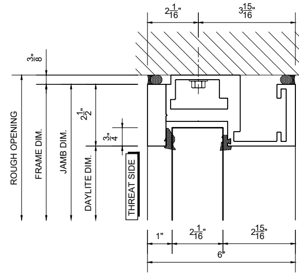
3 HEAD DETAIL SCALE: 3" = 1'-0"
