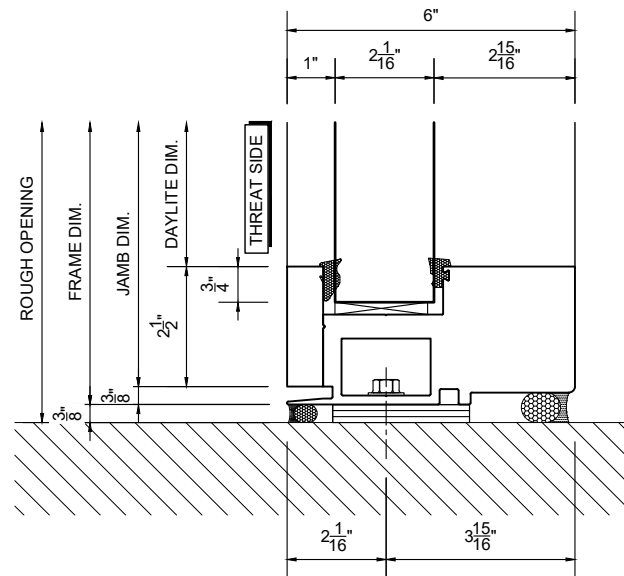
5 SILL DETAIL SCALE: 3" = 1'-0"
