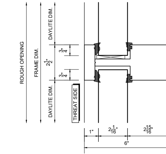
4 INT. HORIZONTAL DETAIL SCALE: 3" = 1'-0"
