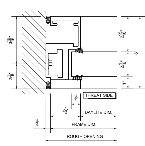
6 JAMB DETAIL SCALE: 3" = 1'-0"
